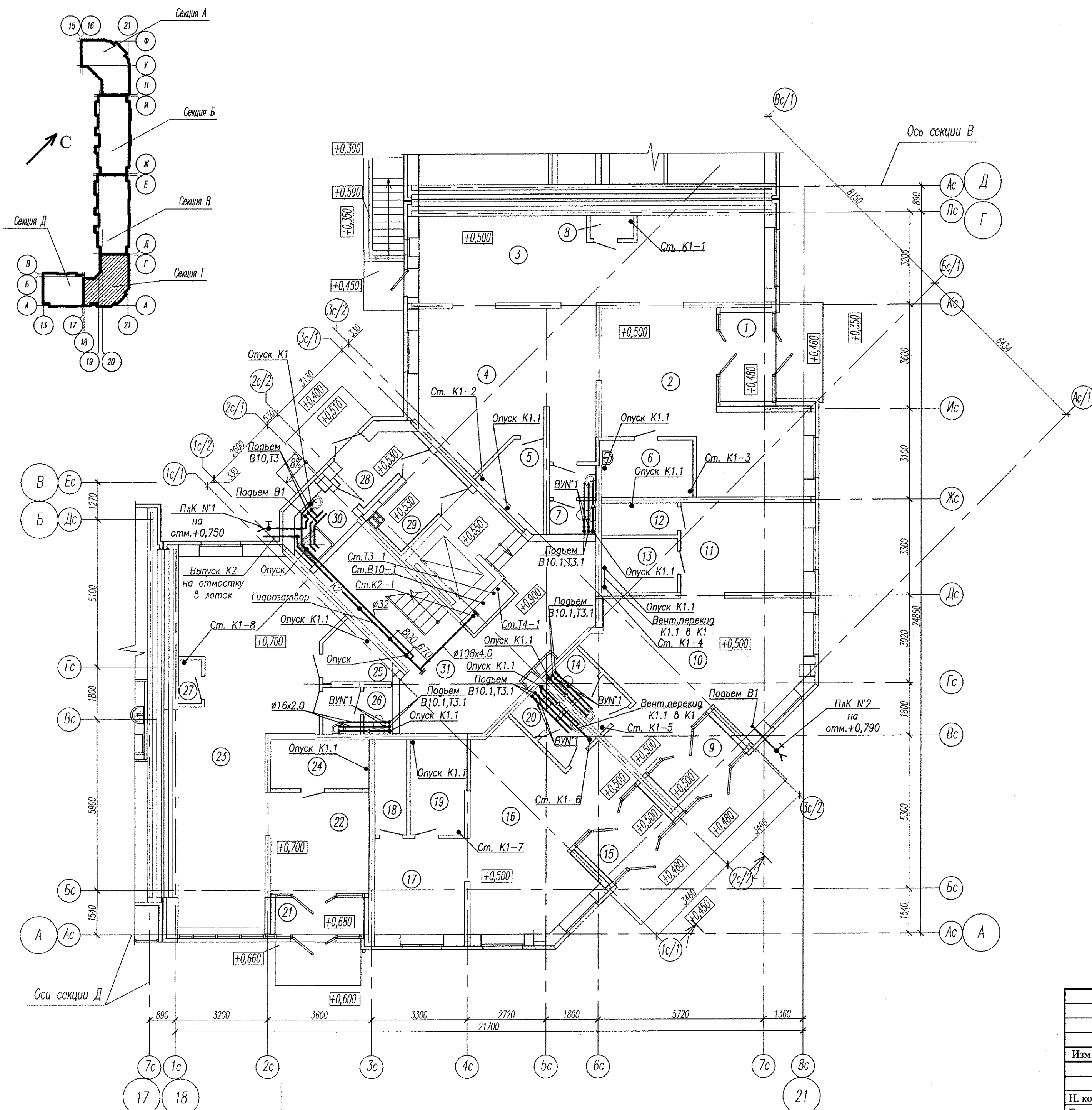
Компоновочная схема дома 1
